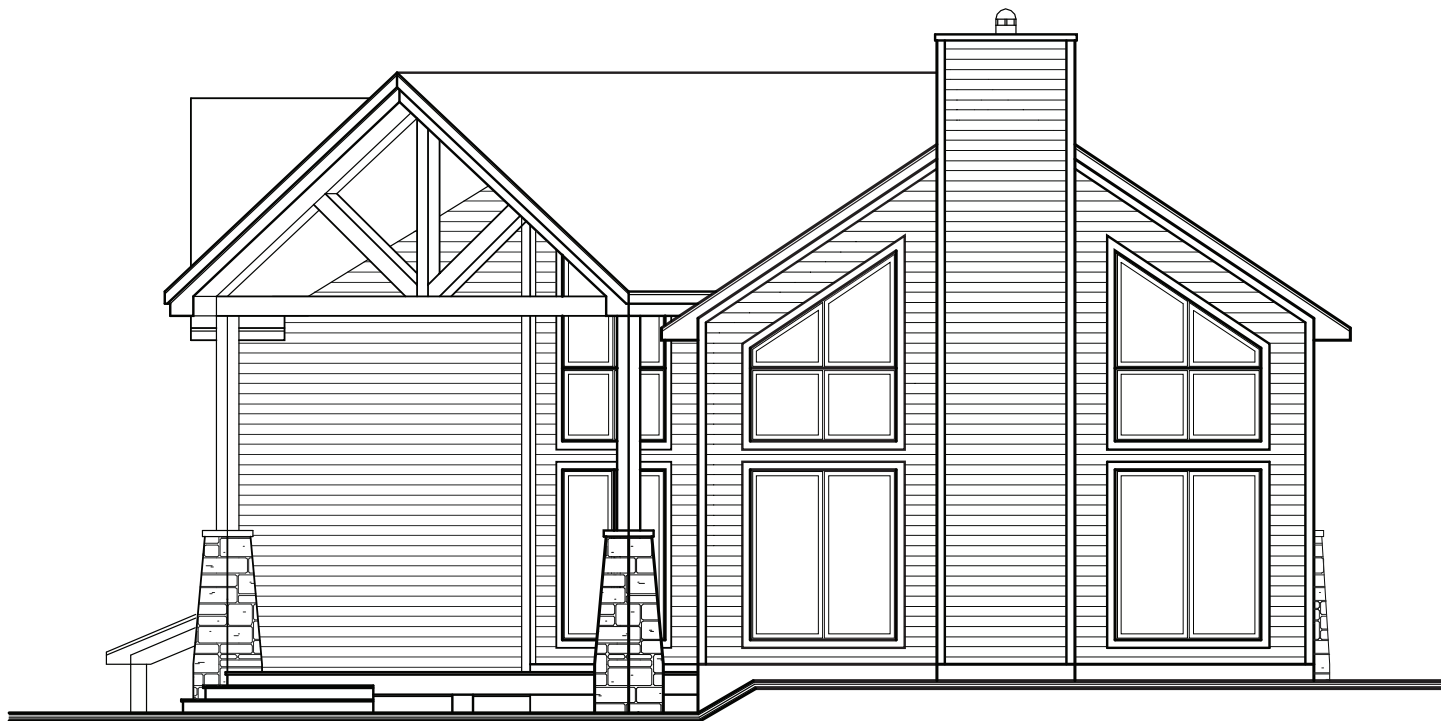
ELEVATION ARRIERE
